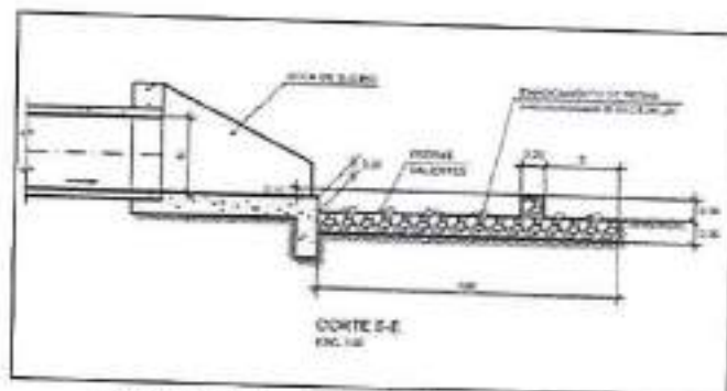
Figura 8.15 – Dissipador de energia
