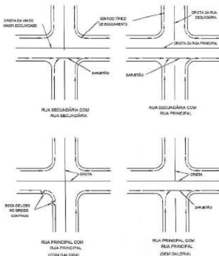
Figura 4.2 – Configurações típicas de cruzamentos em sistema de drenagem
