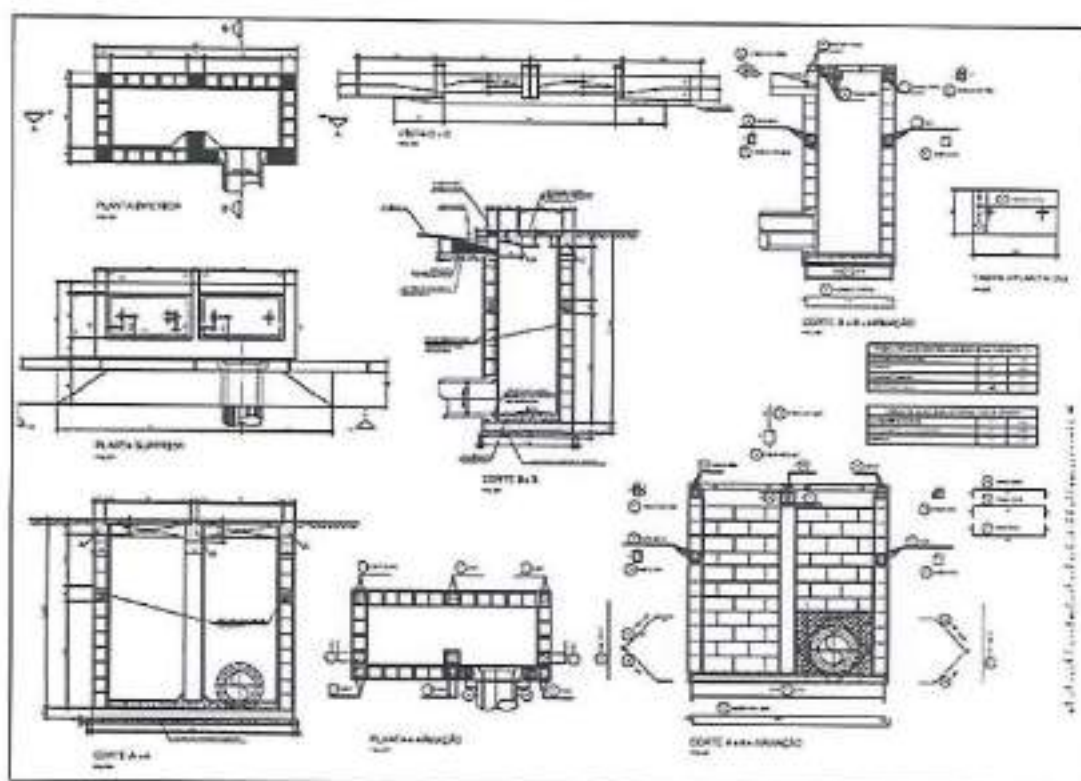
Figura 8.4 – Boca de lobo dupla
