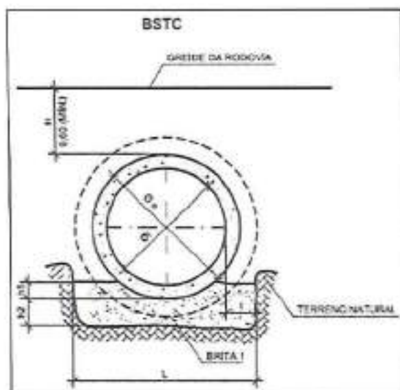
Figura 8.11 – Assentamento de BSTC
