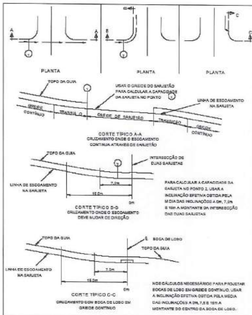
Figura 4.6 – Considerações sobre o projeto de drenagem nos cruzamentos
