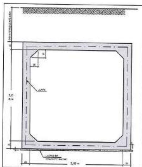
Figura 8.6 – Galeria BSCC 2,00 x 2,00 m
