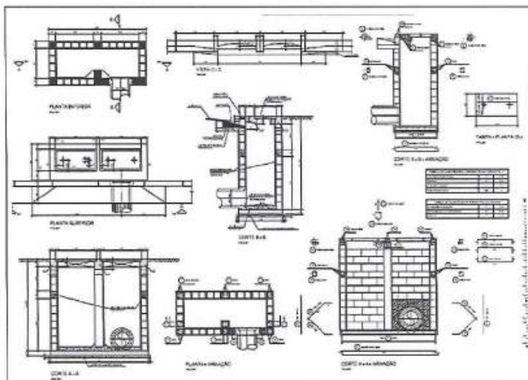
Figura 8.12 – Boca de lobo dupla
